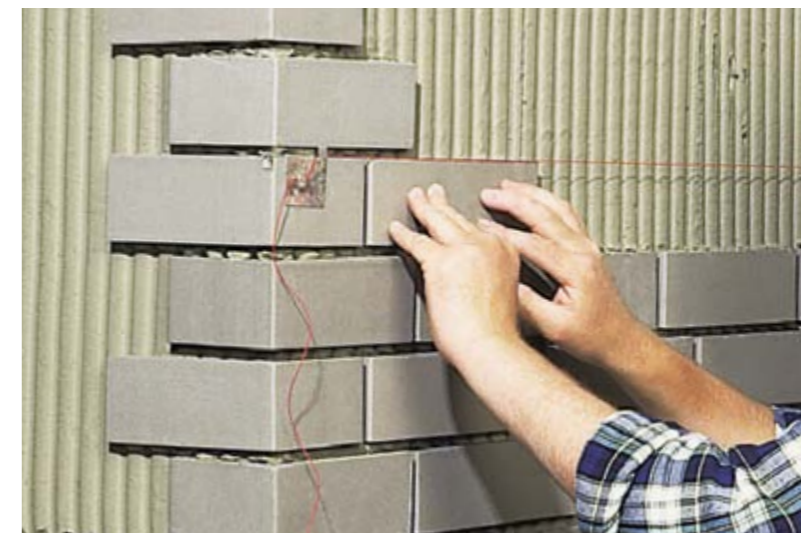
Setzen der Flächenriemchen mit Hilfe einer Schnur.
